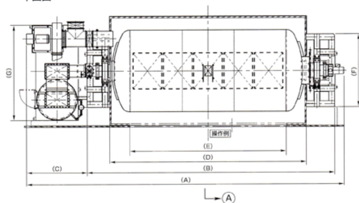
平面図
