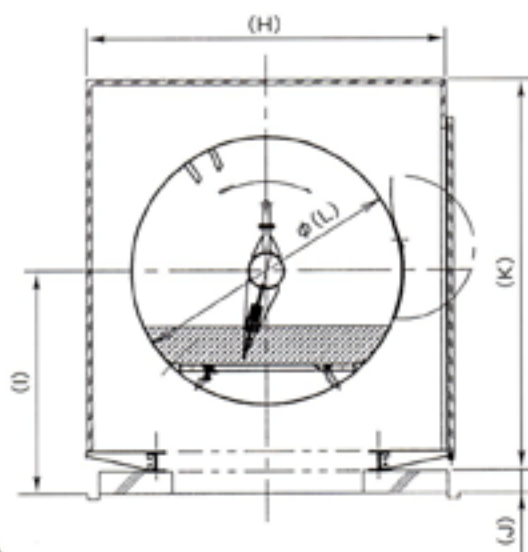
主仕様
